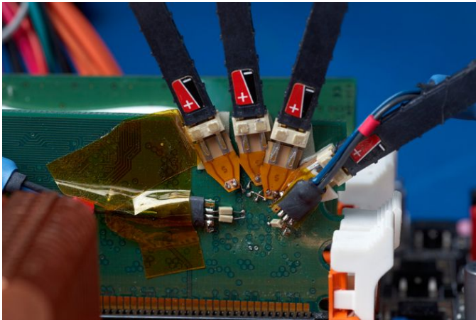
P6780 디퍼렌셜 로직 프로브용으로 설계된 솔더 팁 액세스러리는 좁은 간격의 바이어스 및 미세 회로 구성 요소의 신호에 대한 액세스를 제공합니다.
